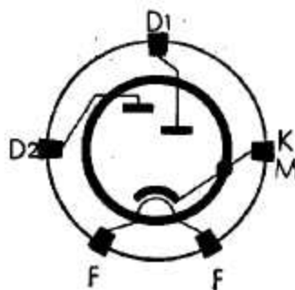
Sockelschaltung
