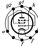
Sockelschaltenschema
