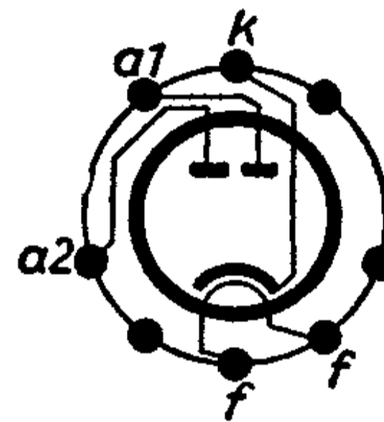
Sockelschaltschema
