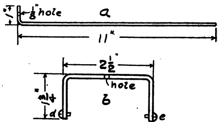
M. E. -FIG. 1-
