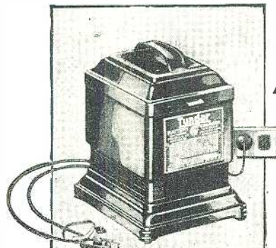
2-ampere Tungar
