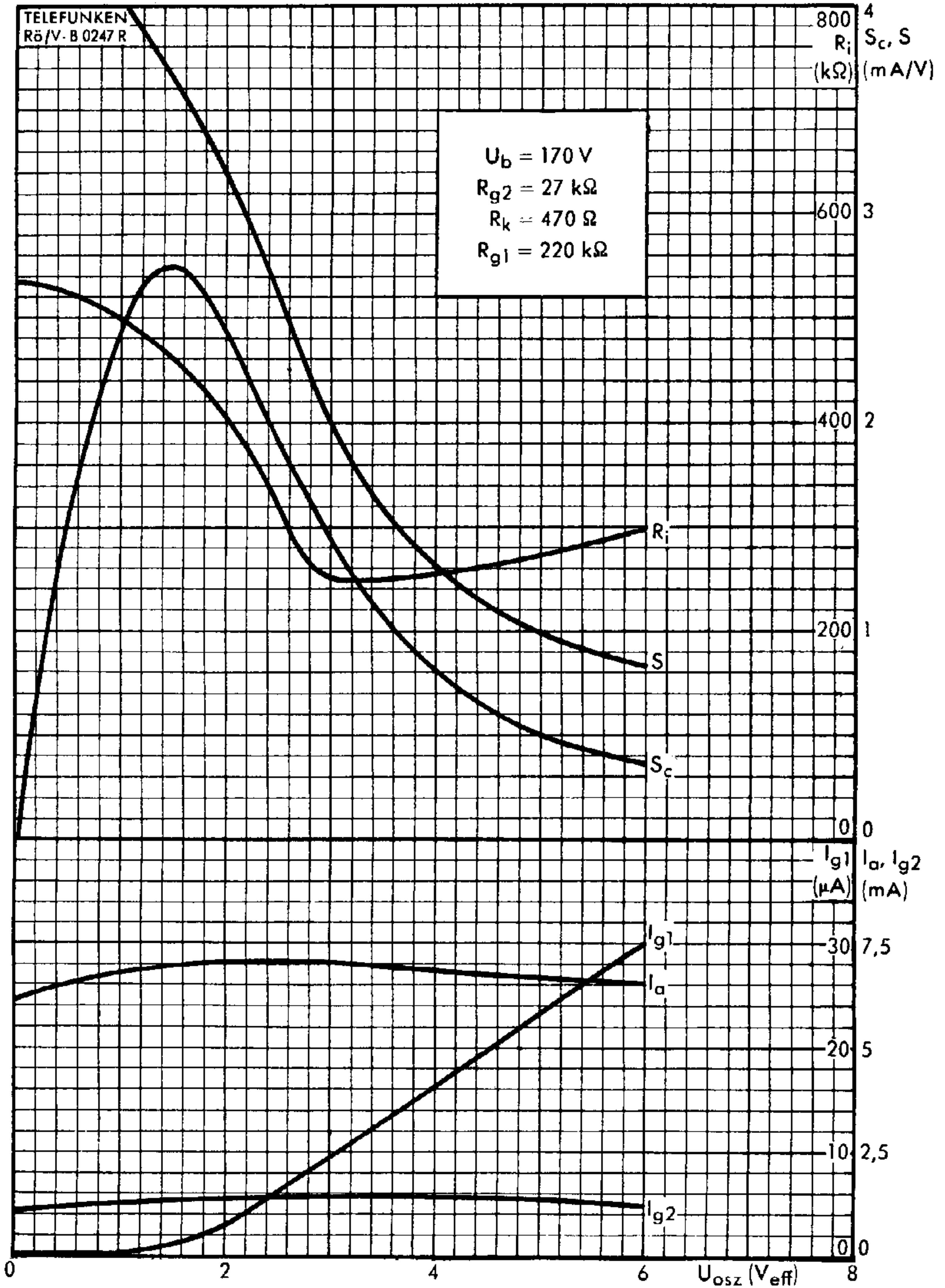
UF 80 als selbstschwingende Mischstufe
