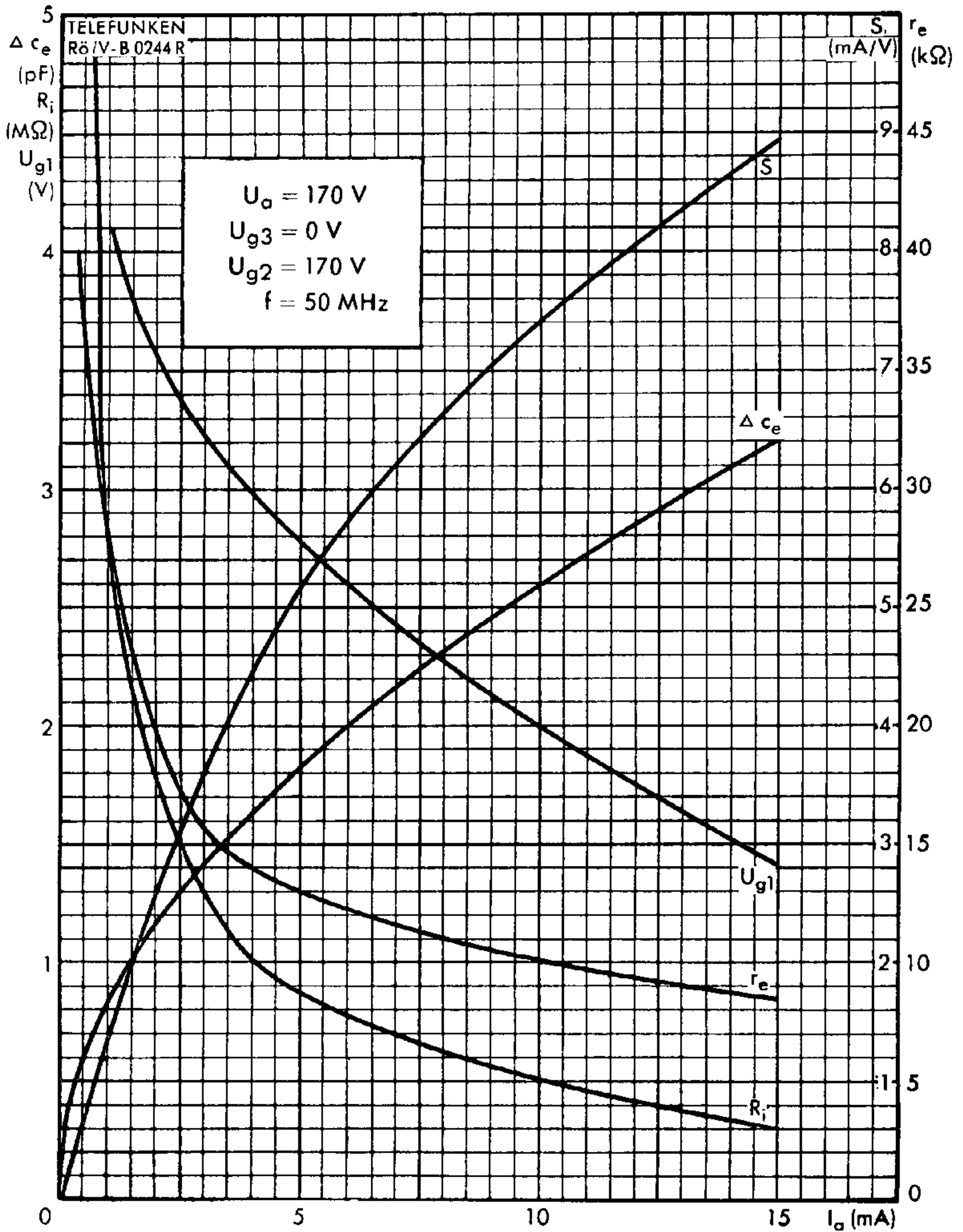
UF 80 als HF-, ZF-Verstärker
