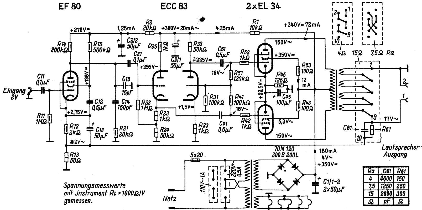
Bild 3. Schaltung des 20-Watt-Hi-Fi-Verstärkers
